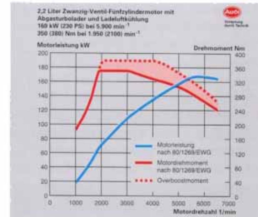
Die Leistungen des 169-kW-Motors mit Overboost-Funktion.
